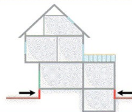
Lábazati fal
